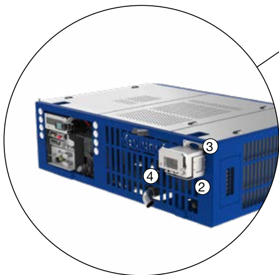
② RICEVITORE RADIO SULL'HOST »ADDRONIC«
